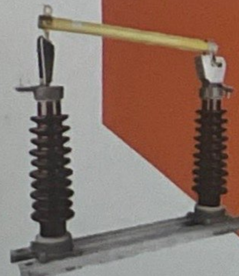
35KV 跌落式熔断器 Drop out fuse Плавильный предохранитель
