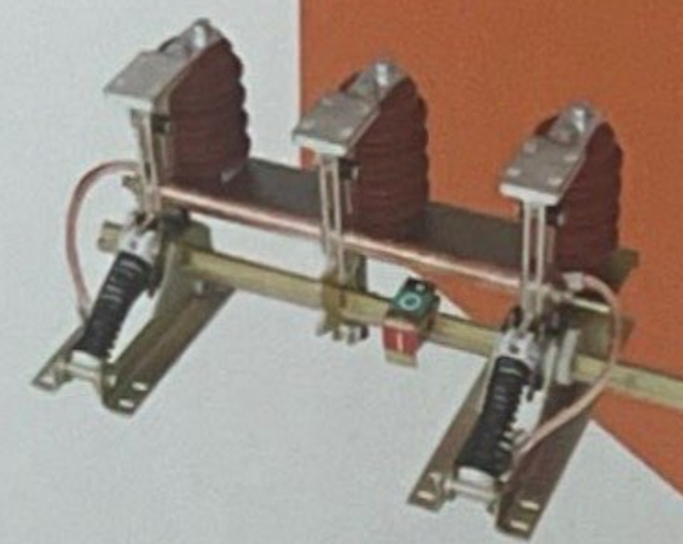
JN15 系列户内高压接地开关 Indoor high-voltage grounding switch Внутренний высоковольтный заземляющий выключатель
