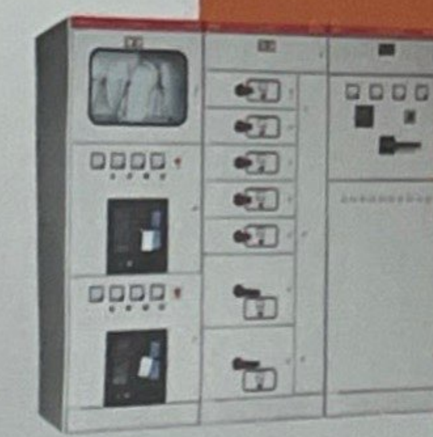
GCK 型低压抽出式成套开关设备 Low-voltage withdrawable switchgear Низковольтные выкатные распределительные устройства
