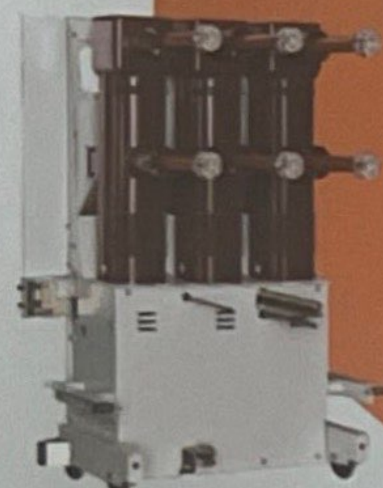
ZN85-40.5/2000-31.5 系列户内高压真空断路器 Indoor high-voltage vacuum circuit breaker Внутривольный вакуумный выключатель
