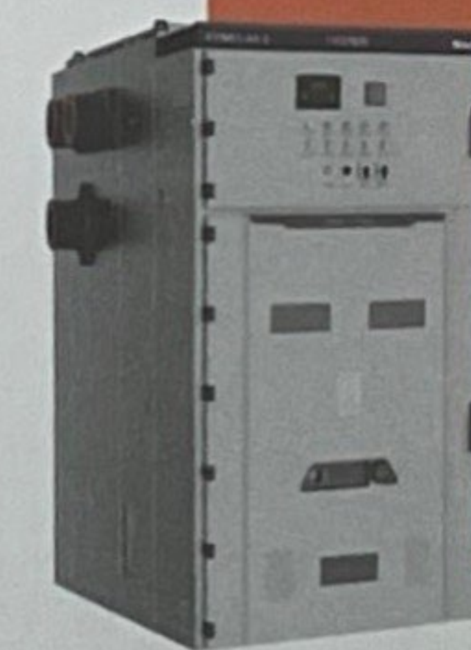
KYN61-40.5Q 型铠装移开式交流金属封闭开关设备 Armoured removable AC metal-enclosed switchgear тип бронированное съемное распределительное устройство переменного тока в металлическом корпусе
