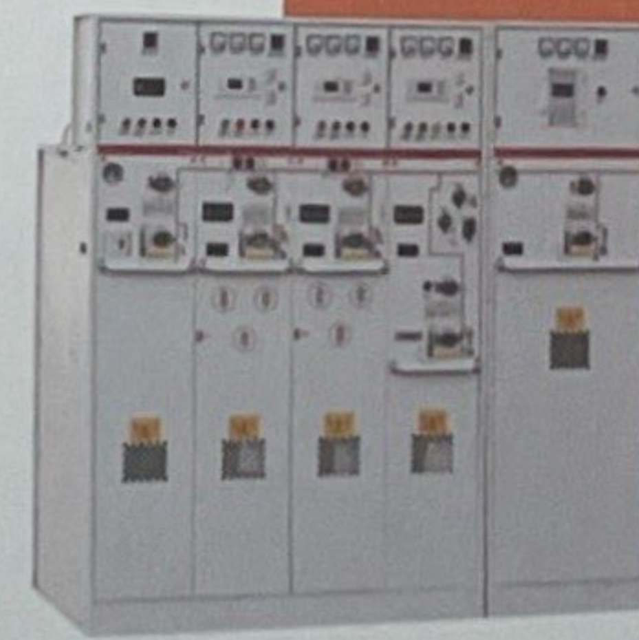
SF6 气体绝缘环网柜 Gas-insulated ring main unit Блок кольцевой основной с элегазовой изоляцией
