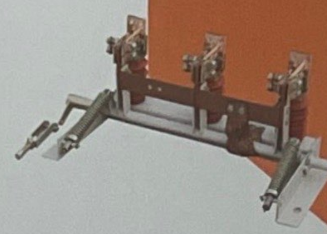
JN14-12 系列户内高压接地开关 Indoor high-voltage grounding switch Внутренний высоковольтный заземляющий выключатель
