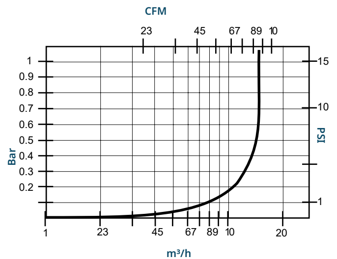
■ Air Discharge
