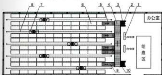
自动化立体仓储平面示意图
