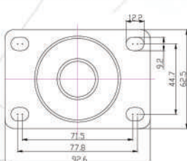
Swivel
