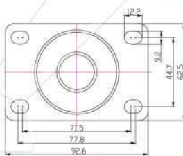
Swivel
