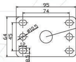
Swivel
