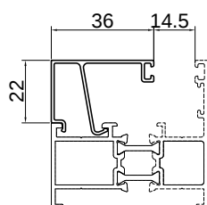
HW55T-B11/ THK. 1.0mm - 0.291 Kg/m
