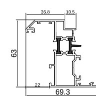
HW55T-B13/ THK. 1.0mm - 0.252 Kg/m
