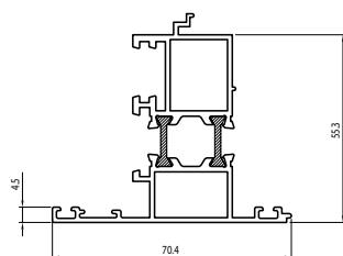
HW55T-B11/ THK. 1.0mm - 0.291 Kg/m
