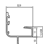
HW68T-C01/ THK. 1.2mm - 0.316 Kg/m
