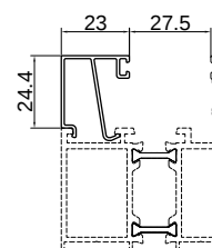
HW55T-B14/ THK. 1.0mm - 0.265 Kg/m
